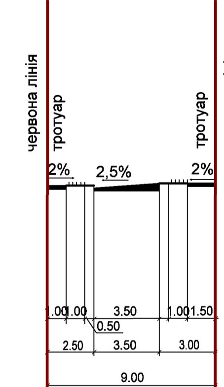
Розріз II-II
