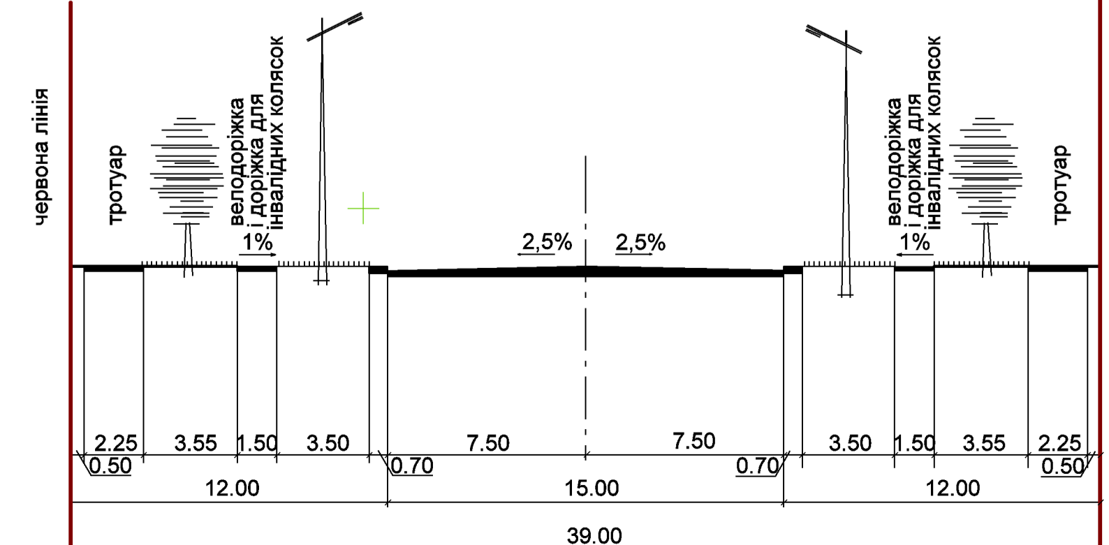
Розріз I-I
